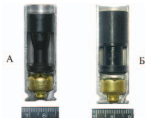
Фото 19. Продольный механический разрез гильзы патрона 18,5х55Т (А) и патрона 18,5х55ТД (Б) производства ООО «Новые оружейные технологии».
