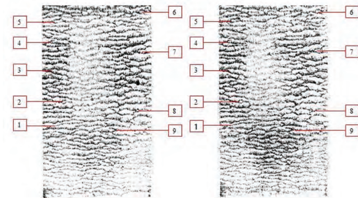
Рис. 2. Следы бумагозахватывающих валиков лазерного принтера Samsung ML-2164 (стрелками и одноименными цифрами отмечены совпадающие частные признаки)
